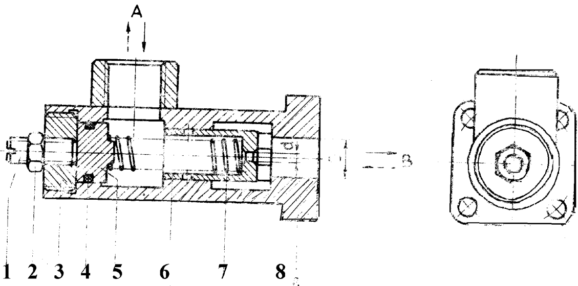
Рис. 23 Нерегулируемый дроссель ДН 12А(1,7Х7,2), ДН 12А(2,2Х7,2)
